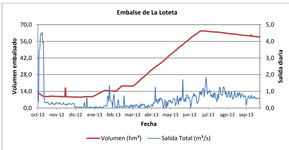
Figura 1. Volumen embalsado y salida durante el año hidrológico 1012-1013.
