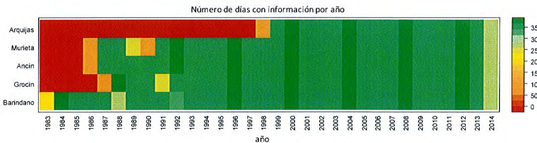
Figura 3: Número de días con datos válidos por año en las series de caudal de Arquijas, Murieta, Ancín, Grocín y Barindano.
