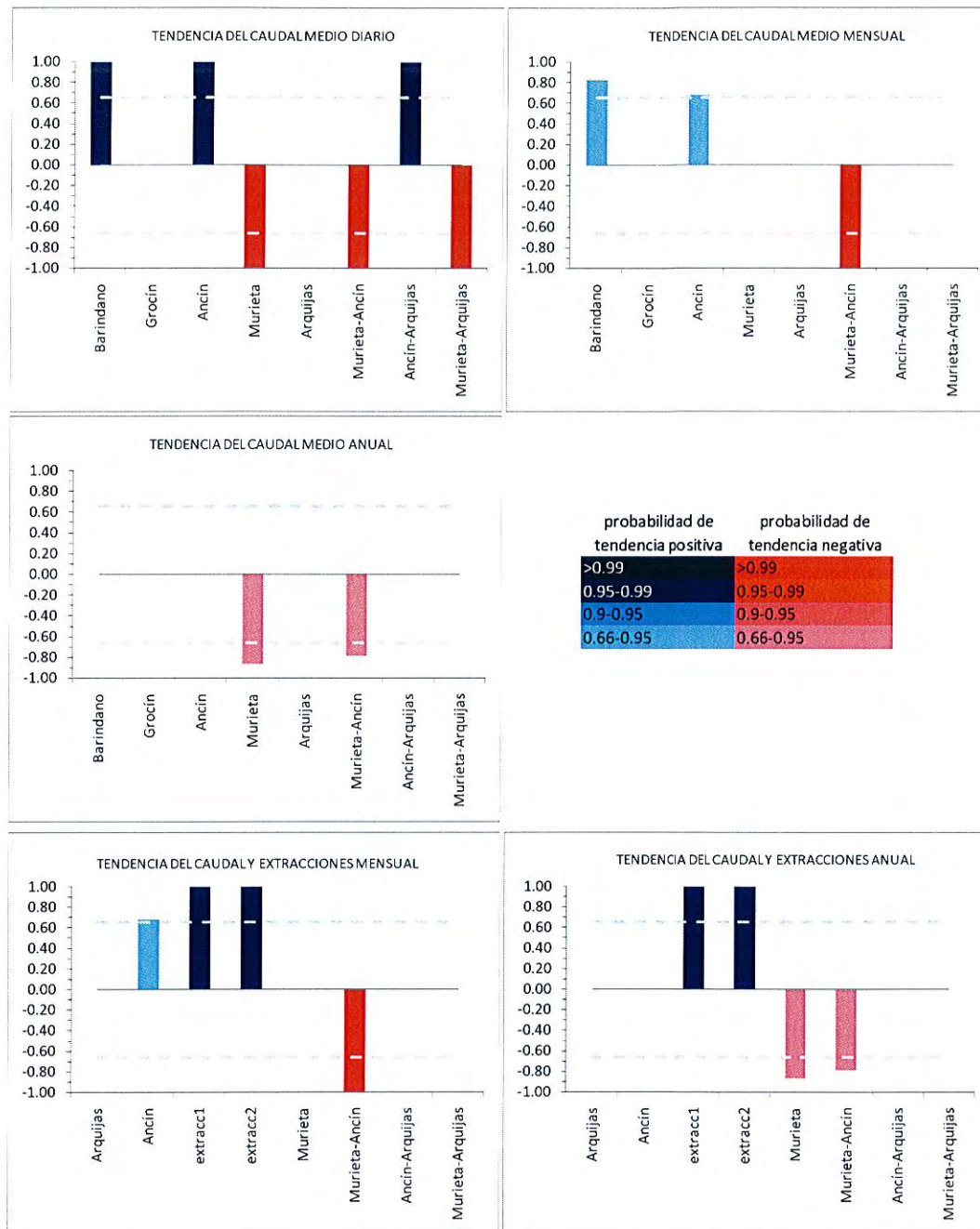
Figura 11: Tendencia de las series de caudal a escala de tiempo diaria, mensual y anual. También se han incluido las tendencias de extracciones junto con las tendencias de caudales del Ega. Solamente se han representado aquellas tendencias con una probabilidad de ocurrencia mayor del 66% ( \pm 0.66 ).
