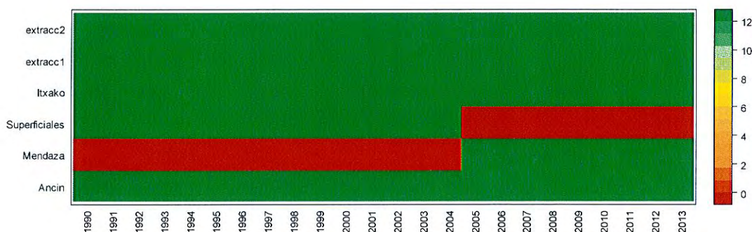
Figura 5: Número de meses con datos válidos para cada año en las series de extracción de agua de la Mancomunidad de Montejurra. Explicación en el texto.
