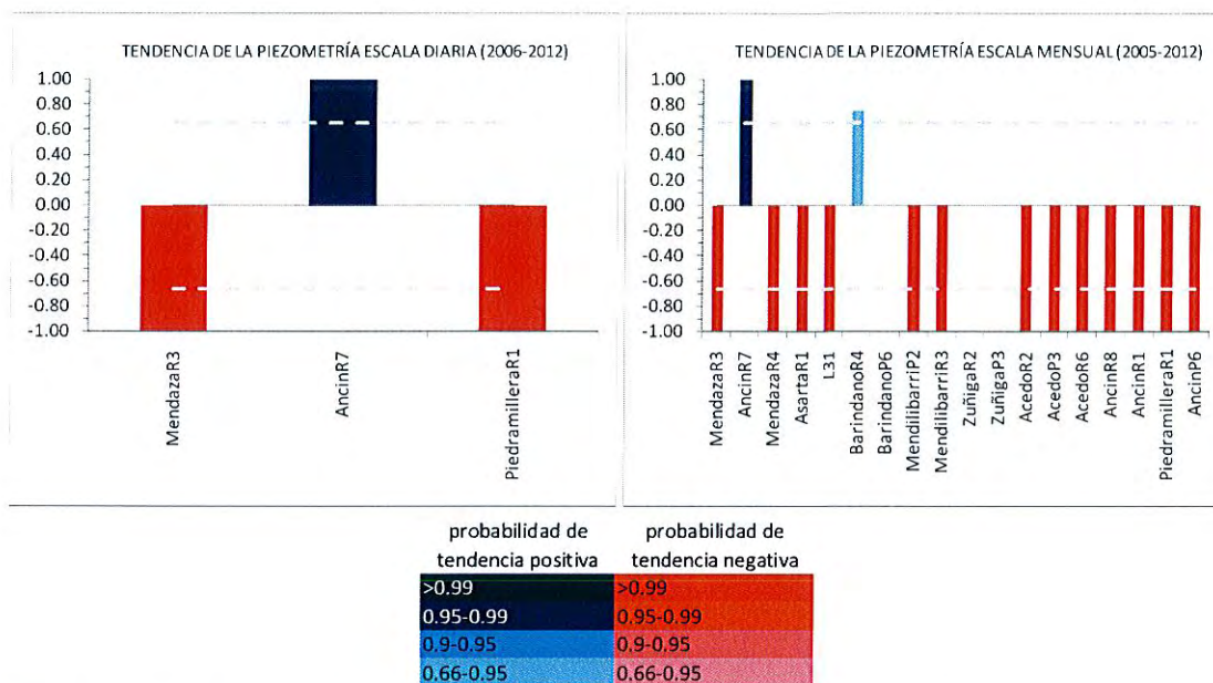
Figura 12: Tendencia de las series de piezometría a escala diaria y mensual. Las series de datos se han considerado desde 2005 hasta 2012 por haber muchas lagunas en los datos anteriores. Solamente se han representado aquellas tendencias con probabilidad de ocurrencia mayor del 66%.
