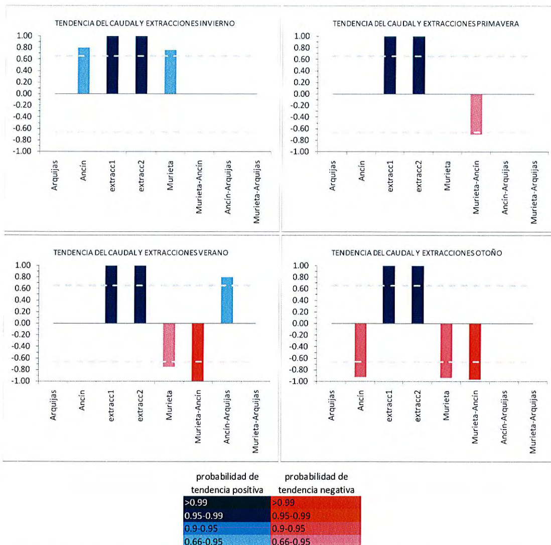
Figura 14: Tendencia estacional de las series de caudal del río Ega y de las extracciones . Solamente se han representado aquellas tendencias con una probabilidad de ocurrencia mayor del 66%.
