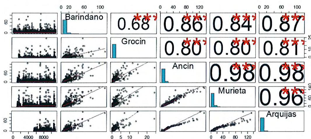
Figura 4: Regresiones y coeficientes de determinación entre las series de caudal analizadas. La primera columna muestra los datos de caudal existentes en cada una de las series. Los gráficos (azul) dispuestos en diagonal muestran los nombres de las estaciones de aforo y los histogramas correspondientes a dichos datos. Los gráficos a la izquierda de esta diagonal se refieren a las regresiones entre cada par de series, y los datos a la derecha de la diagonal a los coeficientes de determinación y la significancia de dichas regresiones. Regresión significativa a nivel: *** = 0.001 ; ** = 0.01 ; * = 0.05 .
