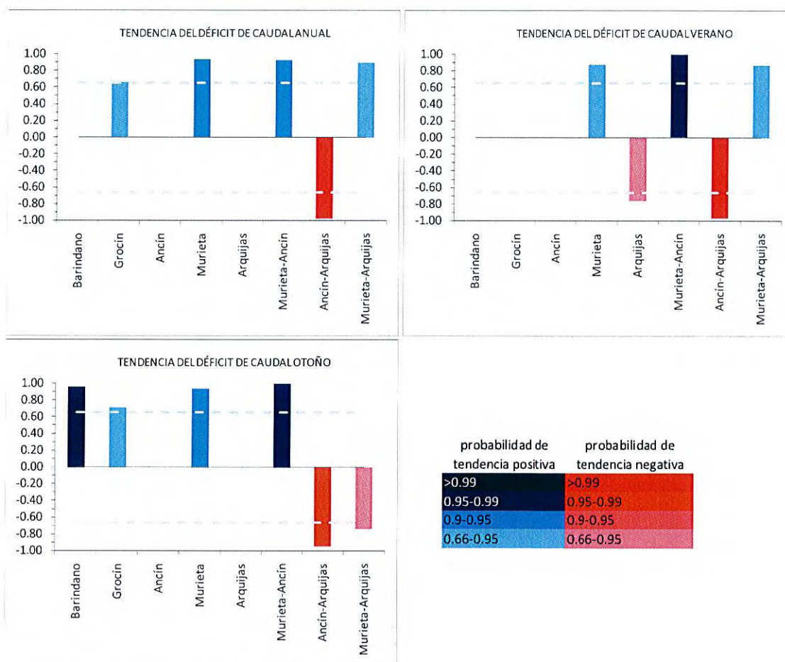
Figura 16: Tendencias del déficit volumétrico de los caudales menores a Q20 a escala anual y para las estaciones de verano y otoño.
