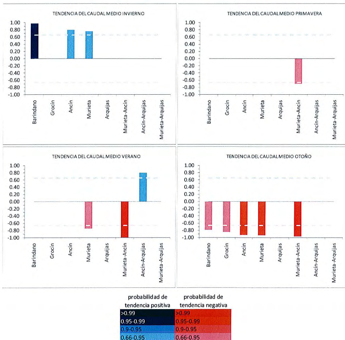
Figura 13: Tendencia de las series de caudal estacional. Solamente se han representado aquellas tendencias con una probabilidad de ocurrencia mayor del 66%.
